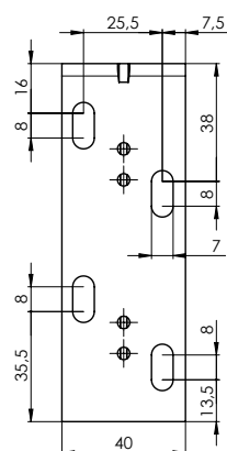
NOSNÍK STAVITELNÝ DVOJITÝ - DLOUHÝ P 003/22 2-01347-XXXX-0
