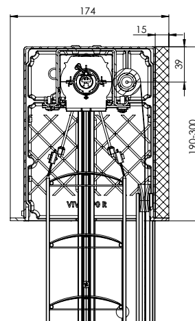
Řez vestavěné samonosné žaluzie Viva (Připraveno pro polystyren z čelní strany + polystyren ze zadní strany)
