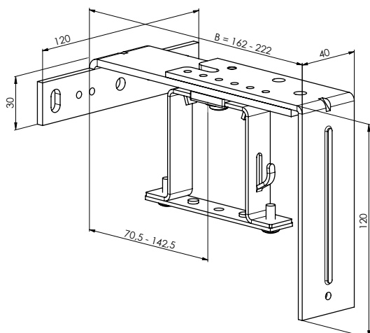
Držák nastavitelný - pevný 162 - 222 mm P 010/34 (2-01603-0000)
