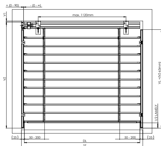
vedení vodicí lištou - kolmá
