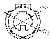
Spojka hřídele P 077/3
