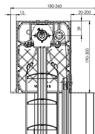
Řez vestavěné samonosné žaluzie Viva (Použití rozšiřující profily) (Připraveno pro polystyren z čelní strany)
