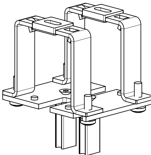
Patka dvojité STS, P002/9
